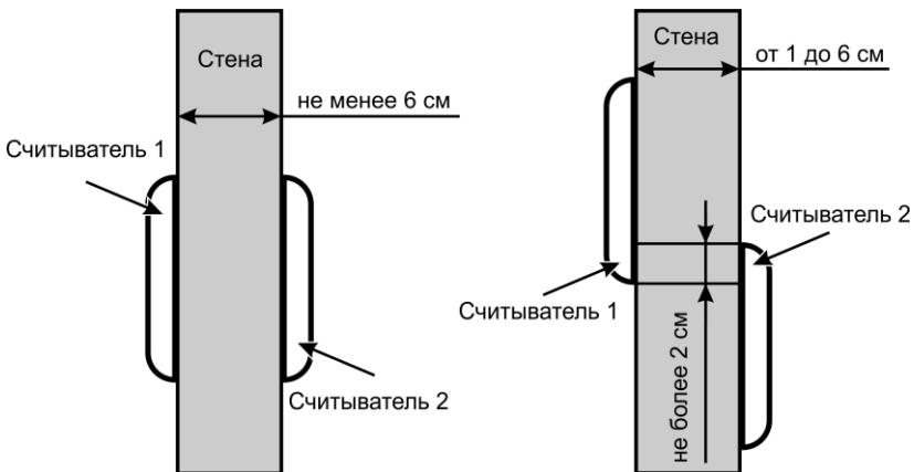
а) Крепление на одном уровне
