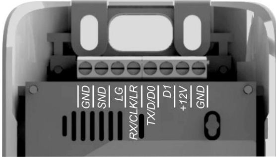
Рисунок 2.4 – Клеммы считывателя
