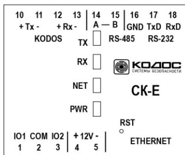
Рисунок 1 – Схема расположения выводов и индикаторов сетевого контроллера СК-Е
