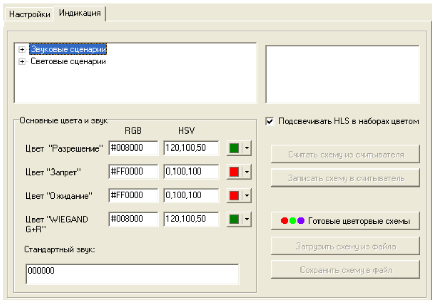
Рисунок 2.10 – Вкладка «Индикация»
