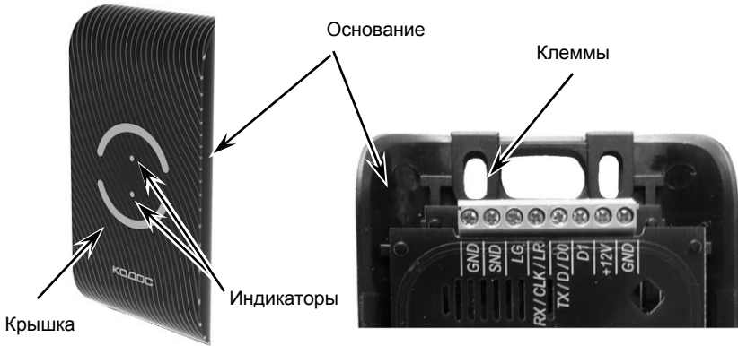
Рисунок 1 – Внешний вид считывателя
