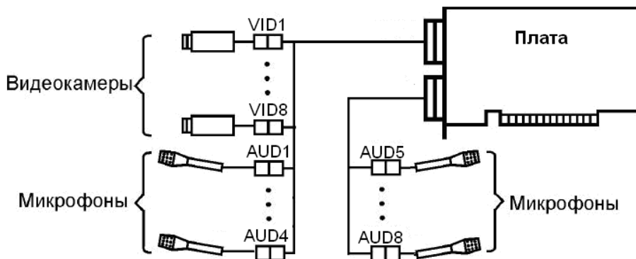
Рисунок 5 – Схема подключения видеокамер
