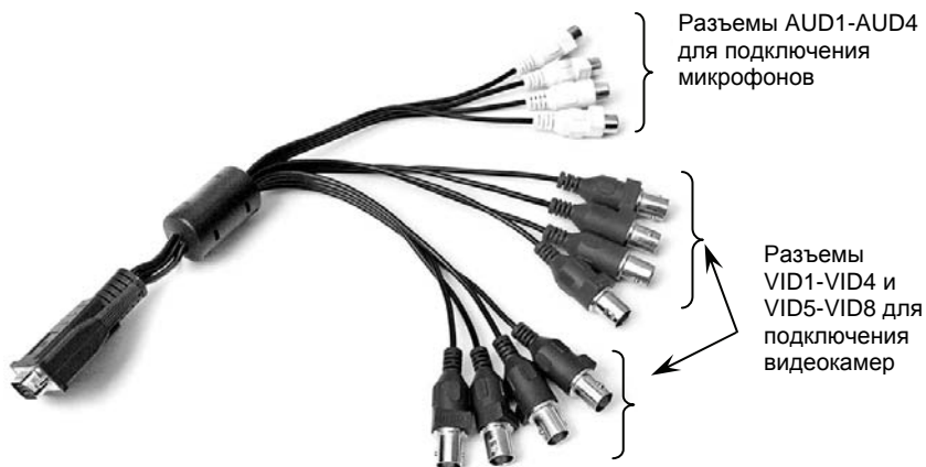
Рисунок 2 – Кабель видеоввода для подключения видеокамер и микрофонов
